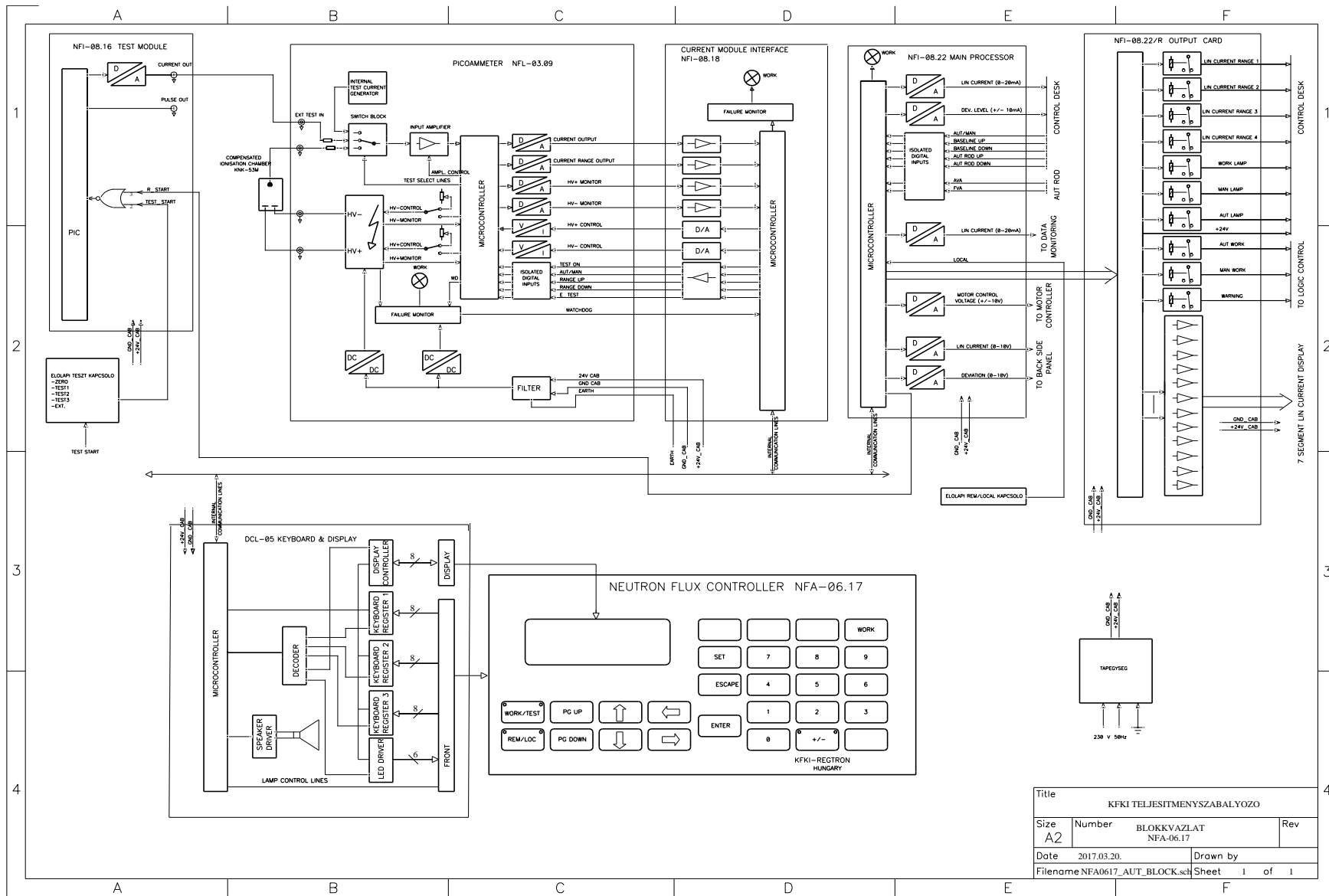
Blokkvázlat
